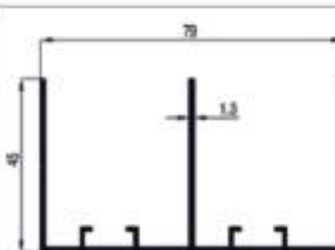
12171 = 0,845 Kg/Mt
