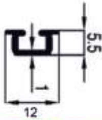
10391 = 0,075 Kg/Mt
