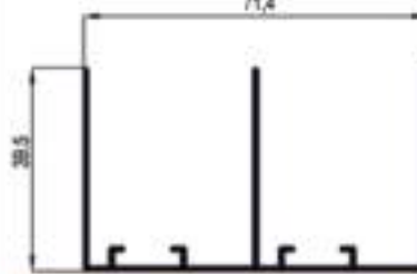
26451 = 0,578 Kg/Mt
