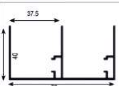
20571 = 0,895 Kg/Mt
