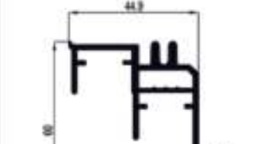
28211 = 0,975 Kg/Mt
