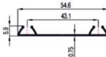
TAP-20091
