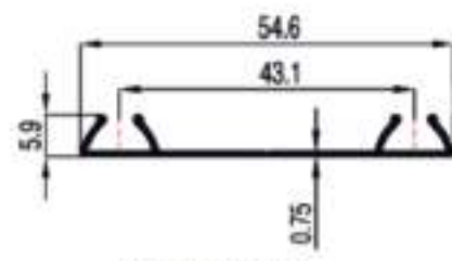
TAP-20091
