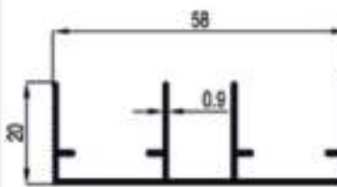
26391 = 0,380 Kg/Mt
