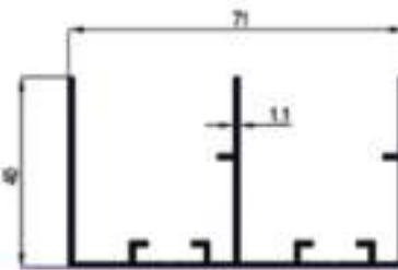
25091 = 0,685 Kg/Mt
