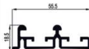
28201 = 0,625 Kg/Mt
