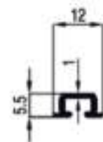
TAP-10391
