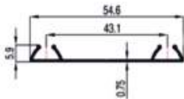
20091 = 0,178 Kg/Mt
