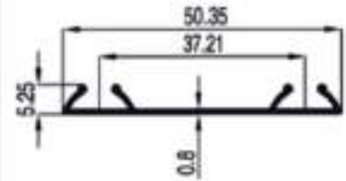
30121 = 0,171 Kg/Mt
