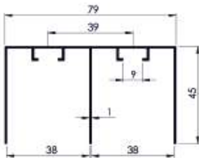
TAP-12171
