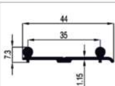
10591 = 0,285 Kg/Mt
