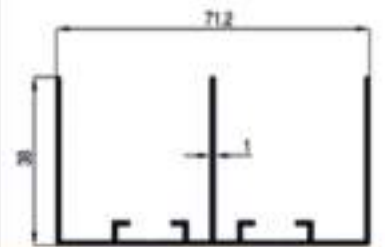
25511 = 0,592 Kg/Mt
